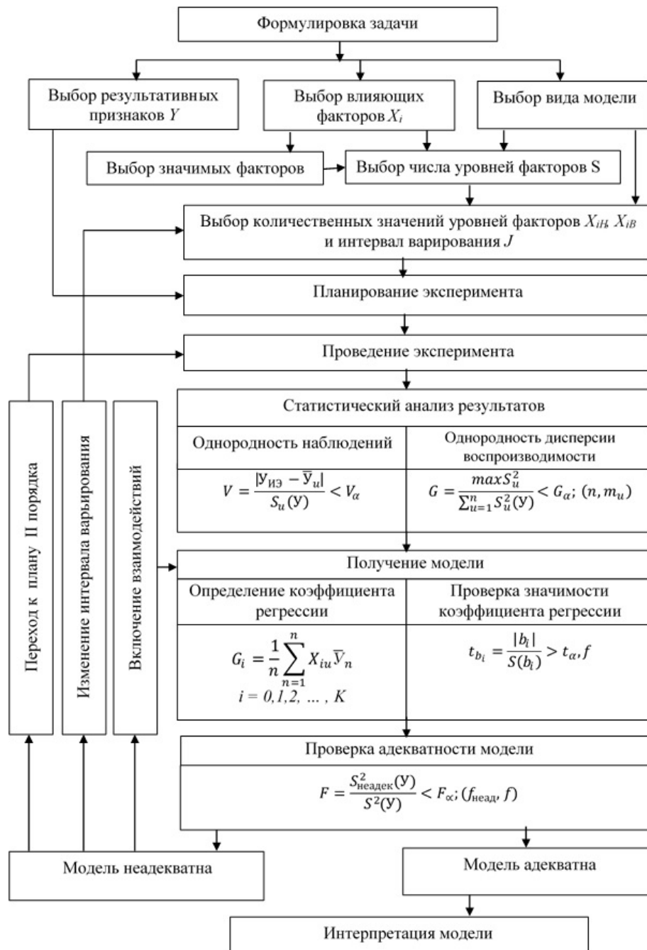
Рисунок 1 – Алгоритм получения математических моделей нормативов технической эксплуатации автомобилей
