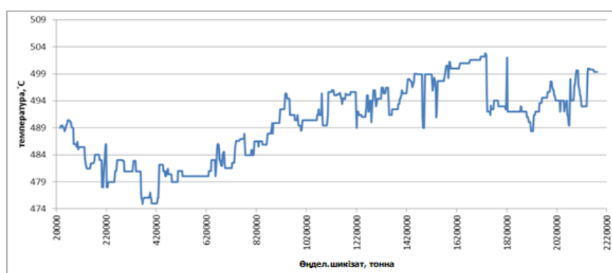
Сурет 2 – Үдеріс температурасының өзгеруі
