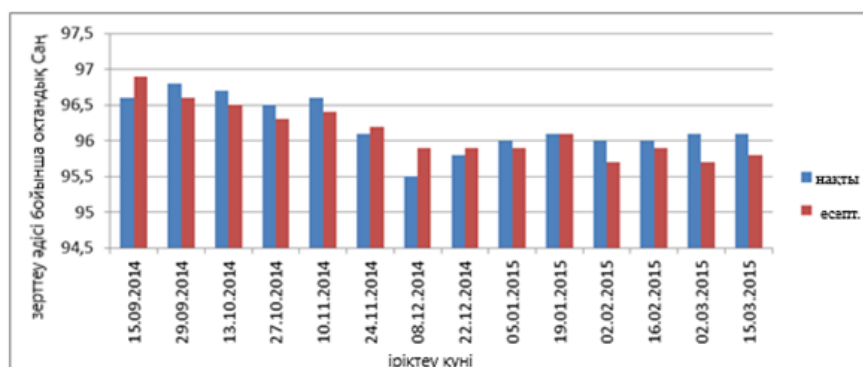
Сурет 1 – Нақты және есептік октандық санын салыстыру
