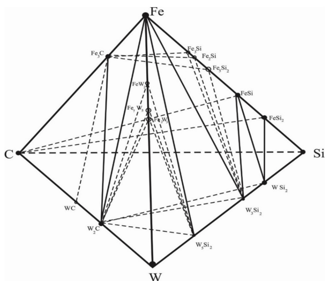
Рисунок 1 – Тетраэдрация металлической системы Fe-W-Si-C
