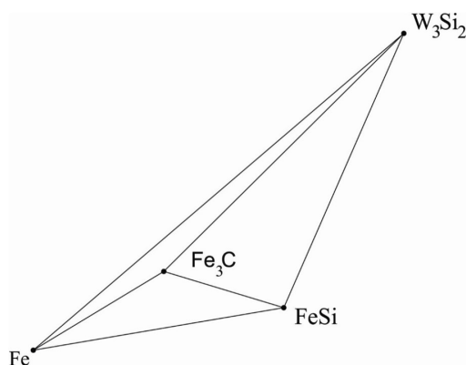
Рисунк 2 – Тетраэдр, моделирующий составы продуктов плавки (ферровольфрама марки ФВ50)
